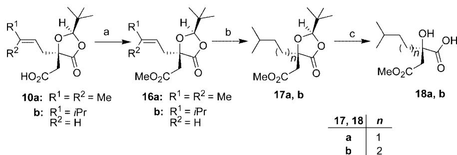
Scheme 7. Reagents: a) MeI, \text{K}_2\text{CO}_3 , DMF, 3 h, quant.; b) \text{H}_2 , \text{PtO}_2 , EtOAc, 95%; c) \text{SiO}_2 , MeOH/ \text{H}_2\text{O} (6:1), 60 °C, 48 h.
